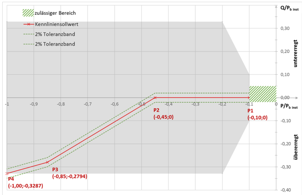
Abb. 13: Anschluss der Erzeugungsanlage an eine Sammelschiene eines MITNETZ STROM-Umspannwerkes mit U_n \leq 20 \text{ kV} und U_n = 30 \text{ kV} , ehemals Bild 10.2
