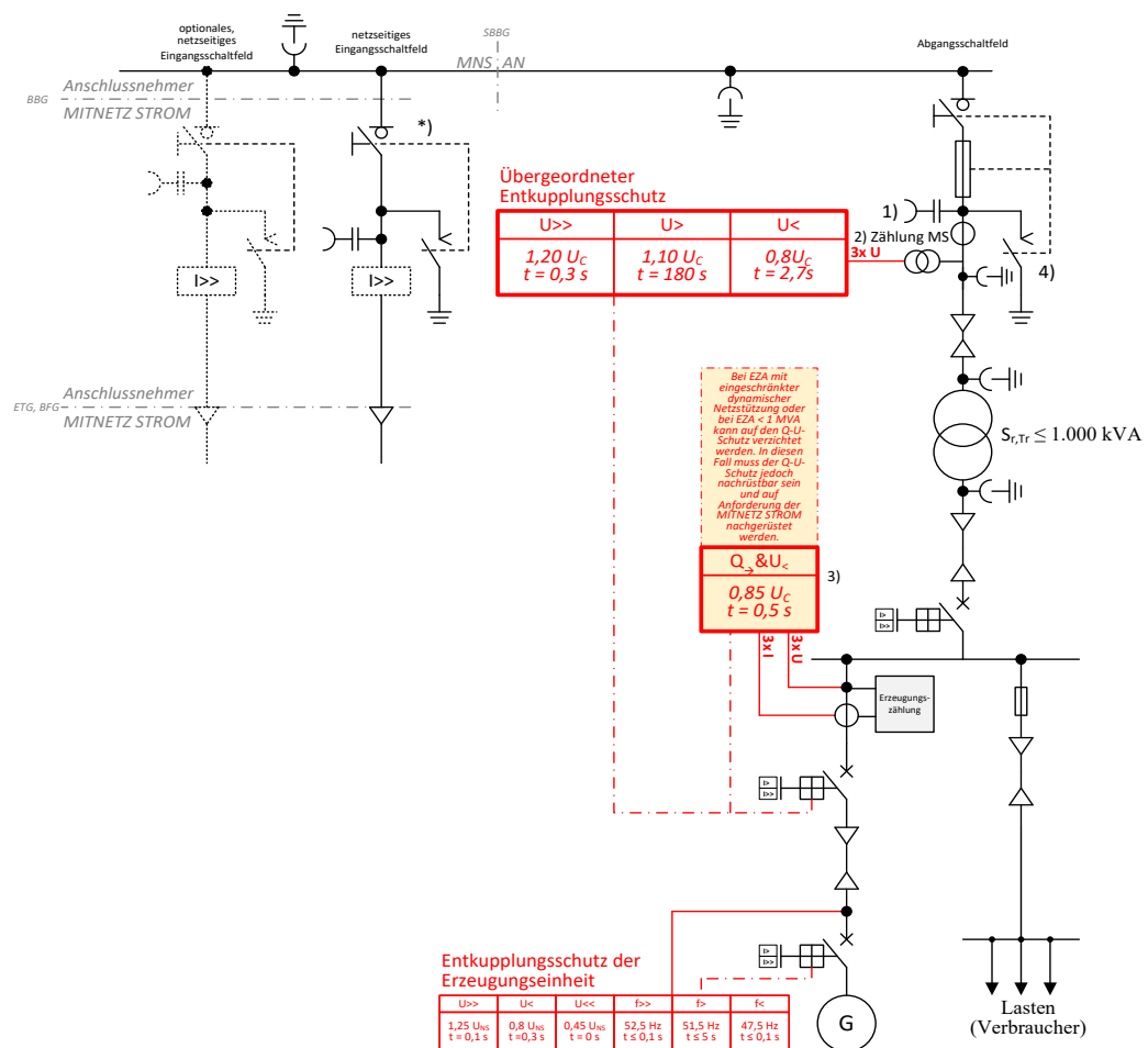
Abb. 33: (ehemals D5a): \leq 20\text{-kV} -Anbindung einer Mischanlage über einen Transformator
