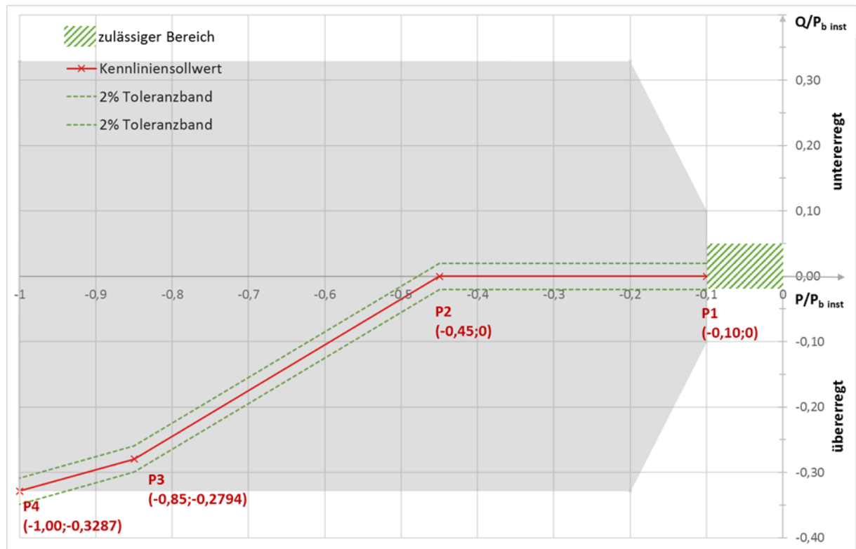
Abb. 13: Anschluss der Erzeugungsanlage an eine Sammelschiene eines EVIP-Umspannwerkes mit U_n \leq 20 kV und U_n = 30 kV, ehemals Bild 10.2
