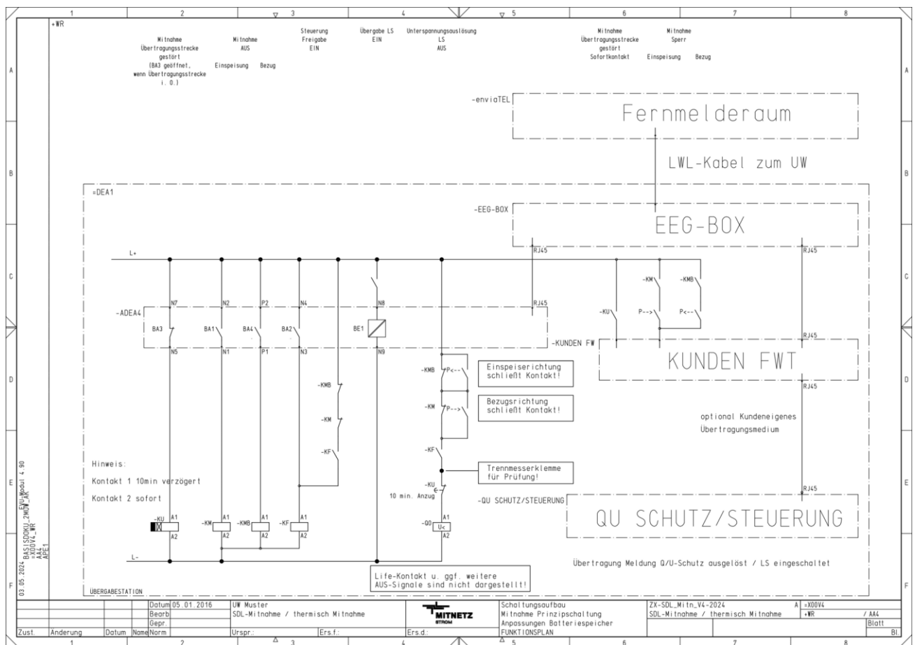
Abb. 52: Schaltungsaufbau der LWL-Kabelverbindung zwischen der Übergabestation und dem EVIP-Umspannwerk (richtungsabhängig)
