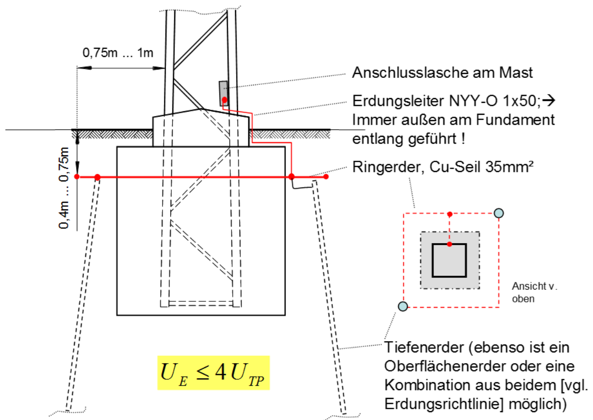
Abb. 7: Standard-MS-Mast-Erdungsanlage
