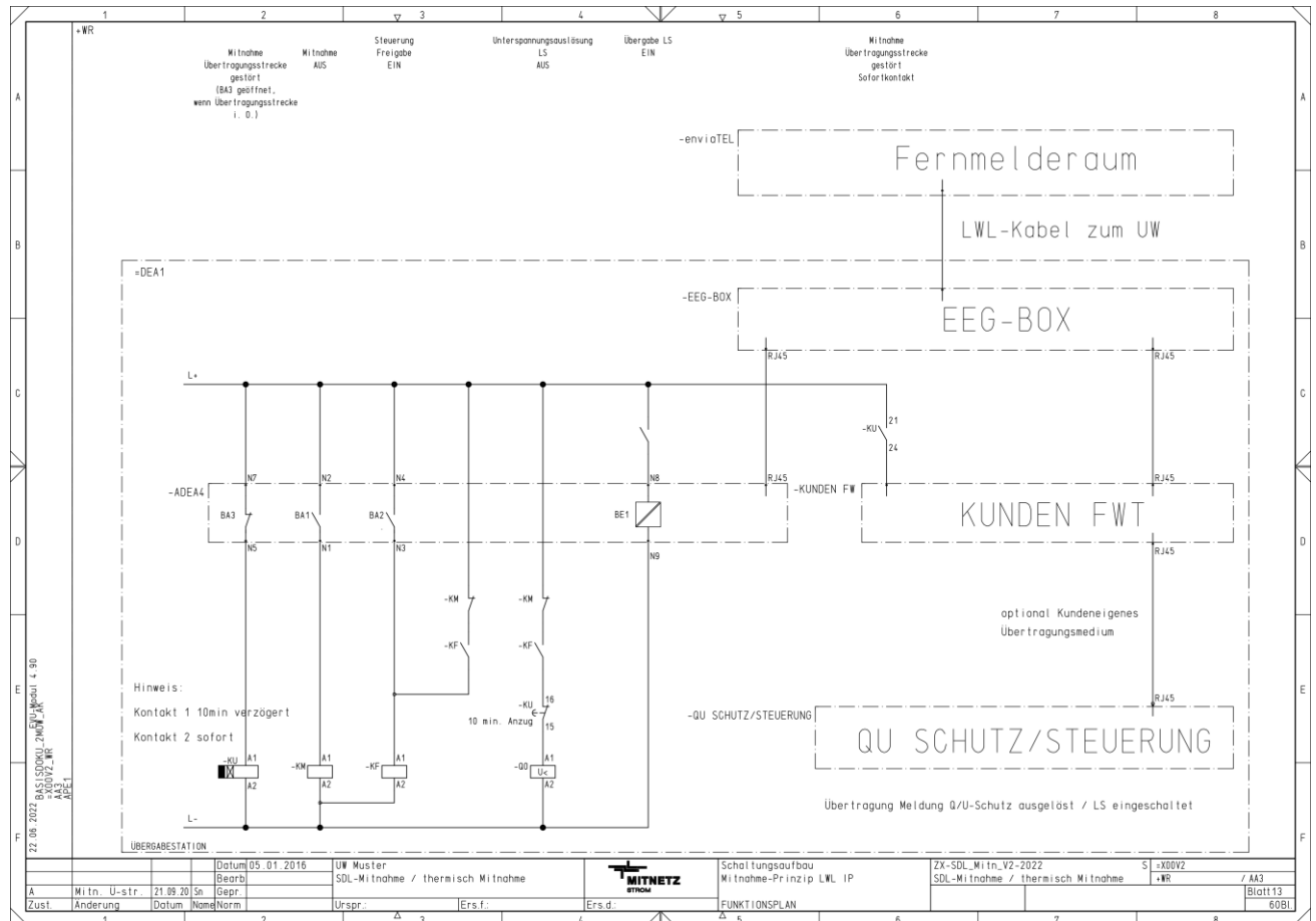
Abb. 51: Schaltungsaufbau der LWL-Kabelverbindung zwischen der Übergabestation und dem EVIP-Umspannwerk (Standardfall)
