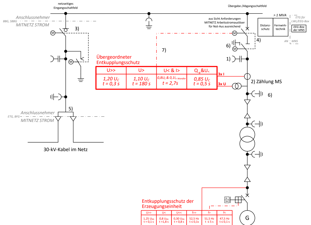
Abb. 36: (ehemals D6): 30-kV-Anbindung einer Erzeugungsanlage im Netz
