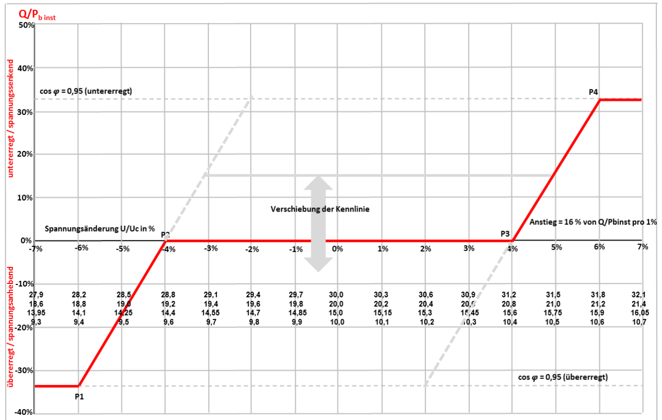
Abb. 15: Standard-Kennlinie Blindleistung mit Spannungsbegrenzungsfunktion, ehemals Bild 10.4
