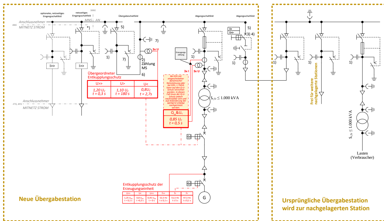
Abb. 34: (ehemals D5d): ≤ 20-kV-Anbindung einer Erzeugungsanlage mit nachgelagerter Station
