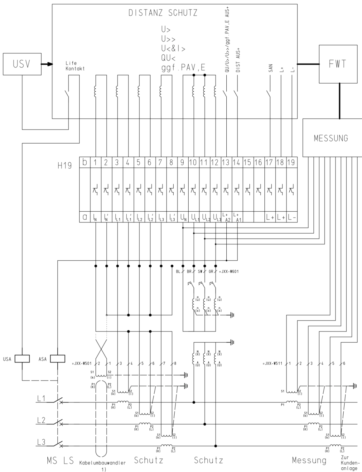
Abb. 48: Wandlerverdrahtung Anbindung Distanzschutz
