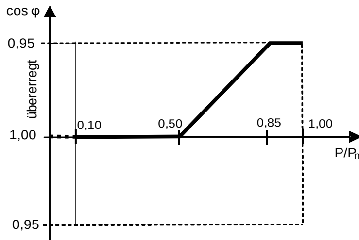
Abb. 53: Anschluss der Erzeugungsanlage an eine MS-Sammelschiene mit U_n \leq 20 kV und U_n = 30 kV (ehemals Bild L.3)
