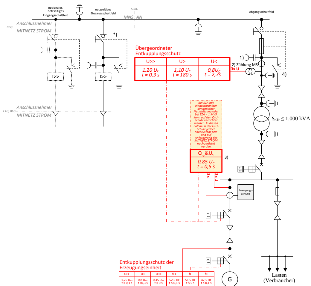
Abb. 31: (ehemals D5a): \leq 20 -kV-Anbindung einer Mischanlage über einen Transformator
