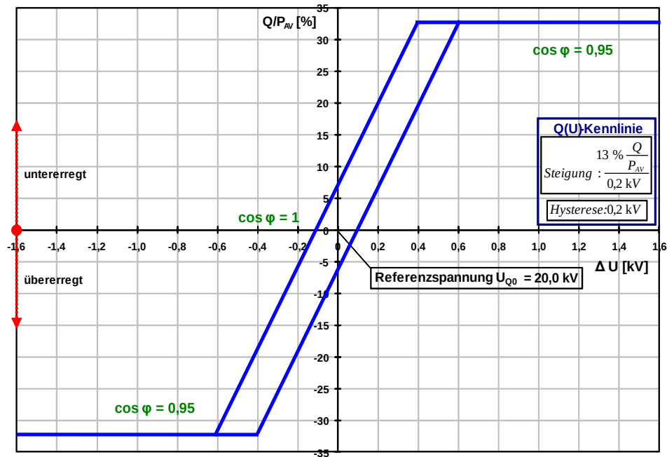
Abb. 51: Q(U)-Kennlinien-Regelung (ehemals Bild L.1)
