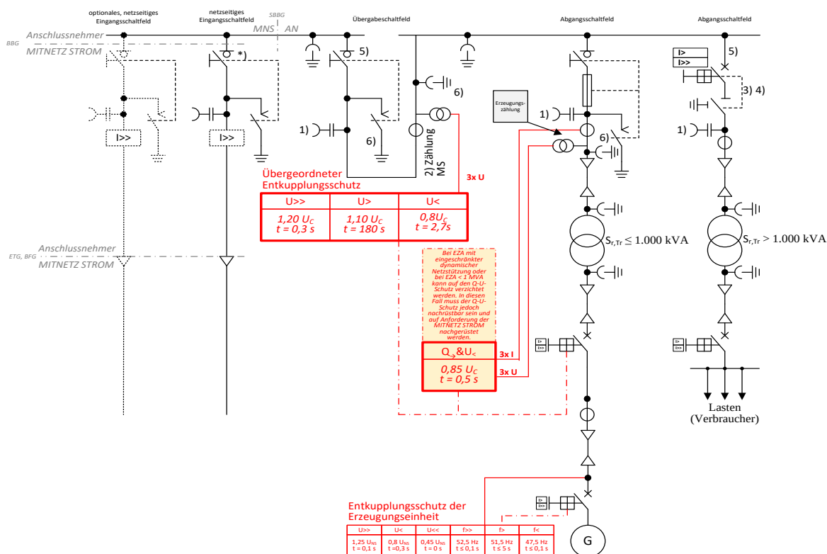
Abb. 32: (ehemals D5b): ≤ 20-kV-Anbindung einer Mischanlage über je einen Transformator für Bezug und Einspeisung
