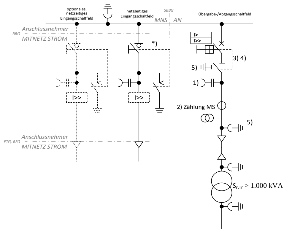
Abb. 22: (ehemals D1b): ≤ 20-kV-Anbindung mit einem Abgangsfeld; Transformator > 1 MVA
