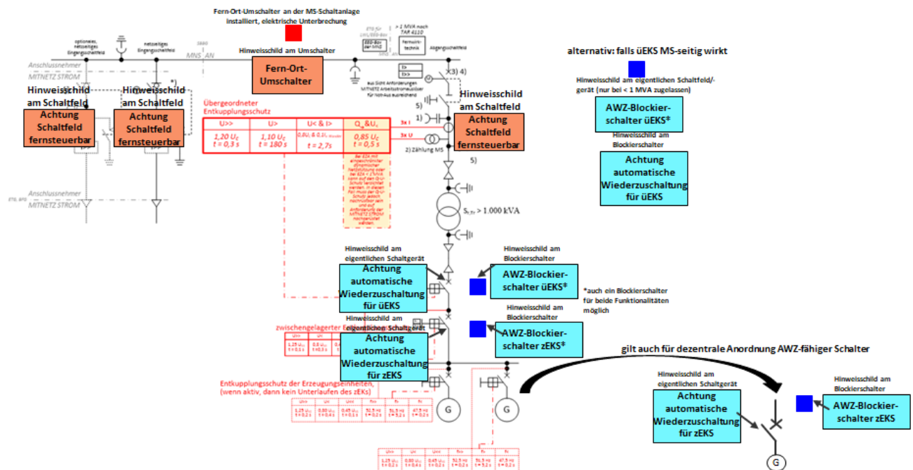
Abb. 5: Beispiel für Kennzeichnung einer fernwirktechnisch angebundenen Übergabestation mit Anbringung von Hinweisschildern
