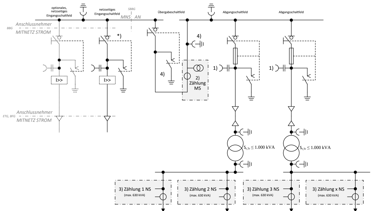
Abb. 23: (ehemals D2a): ≤ 20-kV-Anbindung mit zwei Abgangsfeldern; Transformatoren ≤ 1 MVA mit Übergabe-Lasttrennschalter
