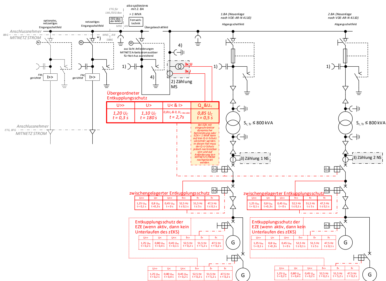
Abb. 30: (ehemals D4e): ≤ 20-kV-Anbindung von zwei Bauabschnitten einer PV-Anlage mit je 750 kVA (spätestens ab 2.BA mit FWT, in diesem Fall im 1.BA mit FRE)
