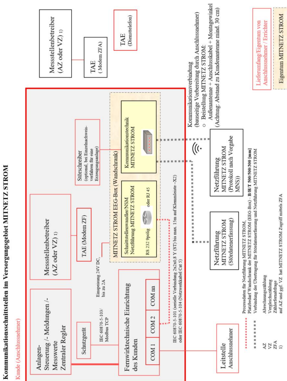
Abb. 18: Kommunikationsschnittstellen
