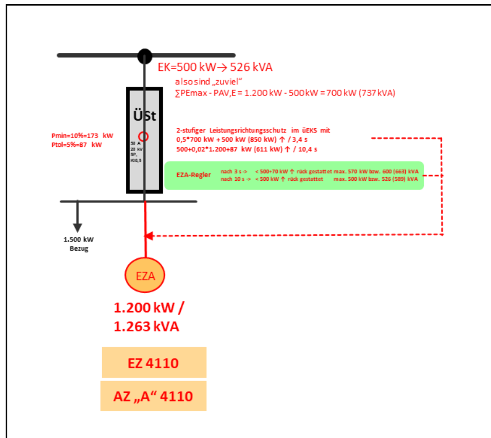
Abb. 17: Beispiel einer P_{AV,E} -Überwachung mit Festlegung der Einstellparameter für den EZA-Regler und die Schutzeinrichtung
