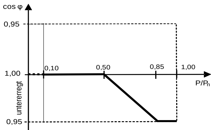
Abb. 54: Anschluss der Erzeugungsanlage im MS-Netz mit U_n \leq 20 kV (ehemals Bild L.4)
