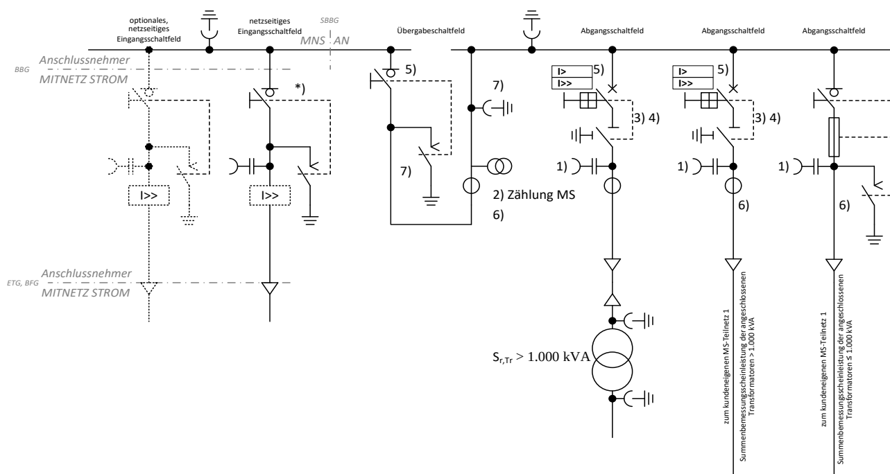
Abb. 24: (ehemals D2b): ≤ 20-kV-Anbindung mit drei Abgangsfeldern (ein Transformator > 1 MVA, zwei Kabelabgangsfelder [kundeneigenes MS-Netz und ein Transformator ≤ 1 MVA bzw. ein Transformator > 1 MVA] mit Übergabe-Lasttrennschalter
