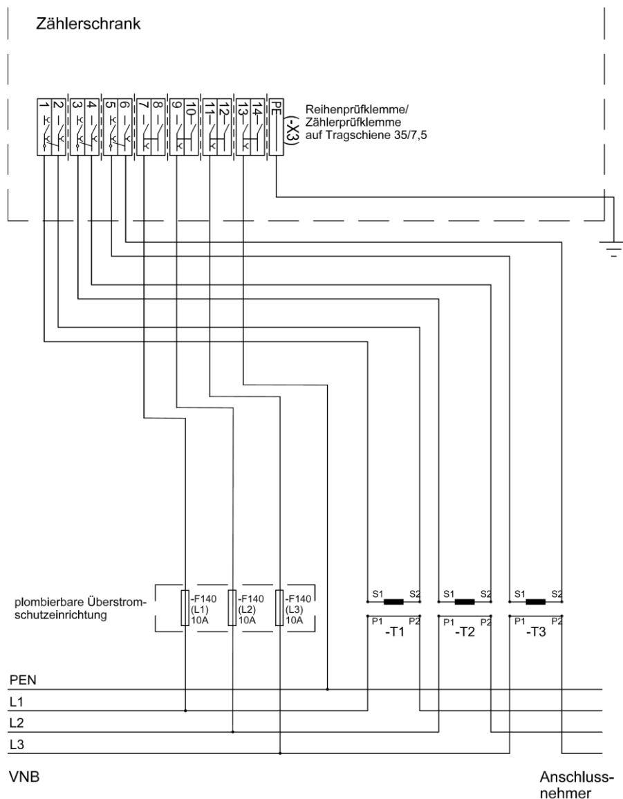
Abb. 43: Messschaltung für die niederspannungsseitige Abrechnungszählung
