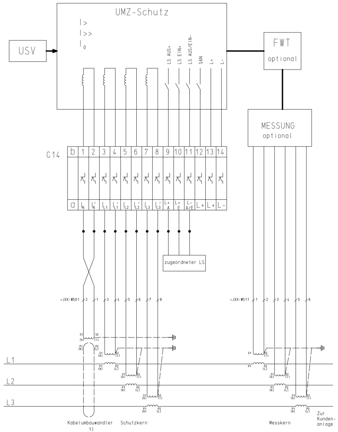
Abb. 45: Wandlerverdrahtung Anbindung UMZ-Schutz
