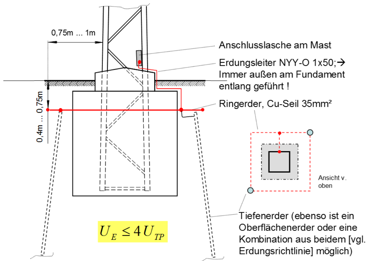
Abb. 7: Standard-MS-Mast-Erdungsanlage
