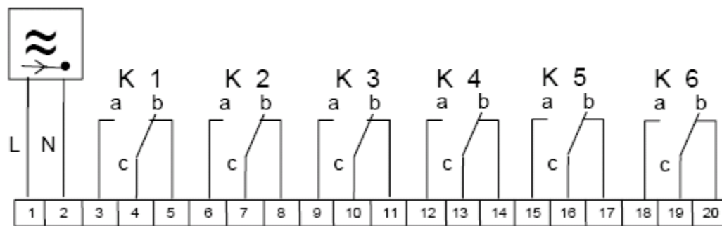
Abb. 16: Relaisplan Funkrundsteuerempfänger
