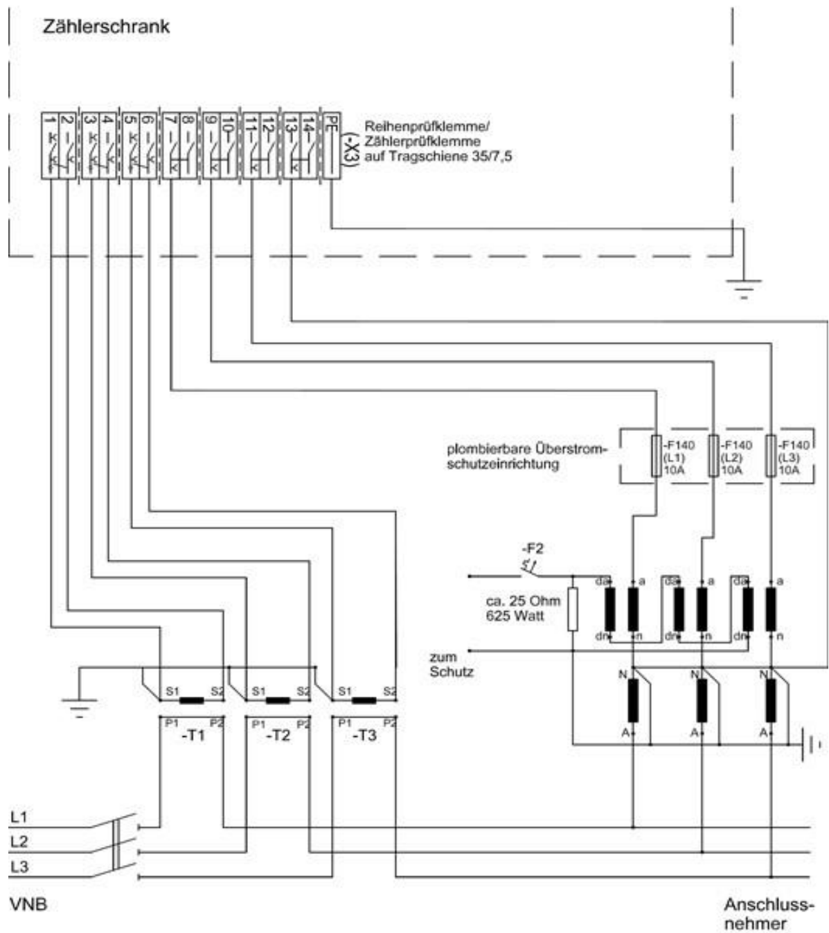
Abb. 42: Messschaltung für die mittelspannungsseitige Abrechnungszählung
