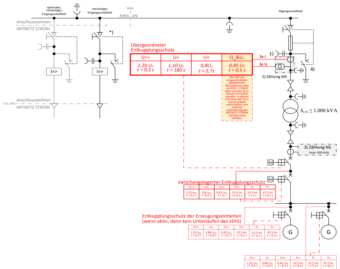
Abb. 28: (ehemals D4c): ≤ 20-kV-Anbindung einer Erzeugungsanlage ≤ 1 MVA
