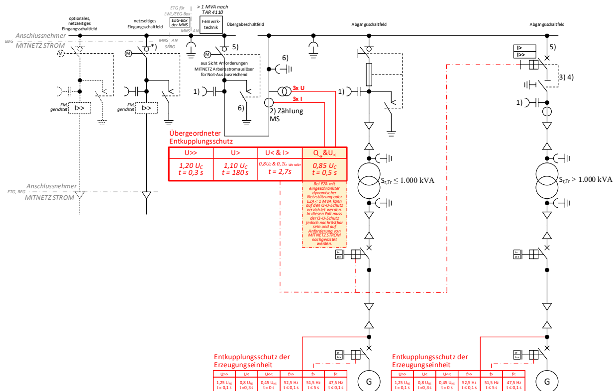
Abb. 26: (ehemals D4a): ≤ 20-kV-Anbindung von zwei Erzeugungseinheiten (1x > 1MVA, 1x ≤ 1MVA) über jeweils einen Transformator
