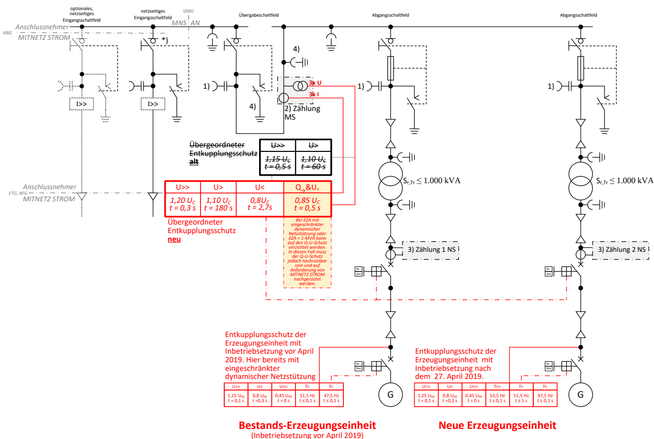
Abb. 27: (ehemals D4b): ≤ 20-kV-Anbindung von zwei Erzeugungseinheiten (Bestands-Erzeugungseinheit; neue Erzeugungseinheit)
