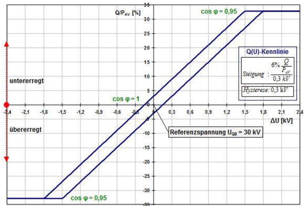
Abb. 52: Q(U)-Kennlinien-Regelung (ehemals Bild L.2)
