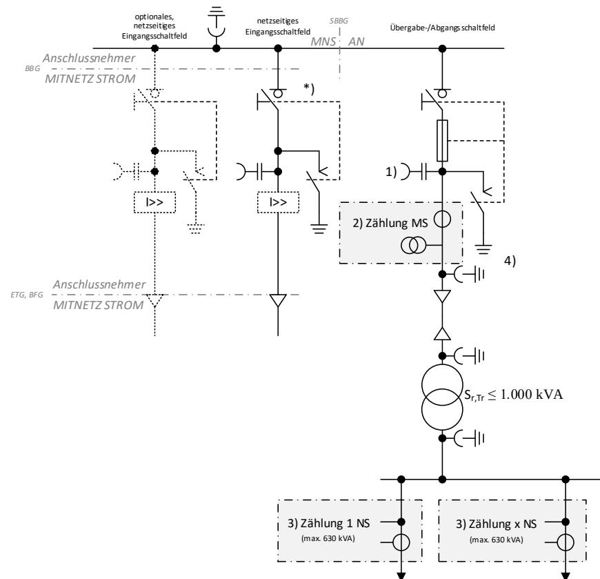
Abb. 21: (ehemals D1a): \leq 20 -kV-Anbindung mit einem Abgangsfeld; Transformator \leq 1 MVA (z.B. 630 kVA)
