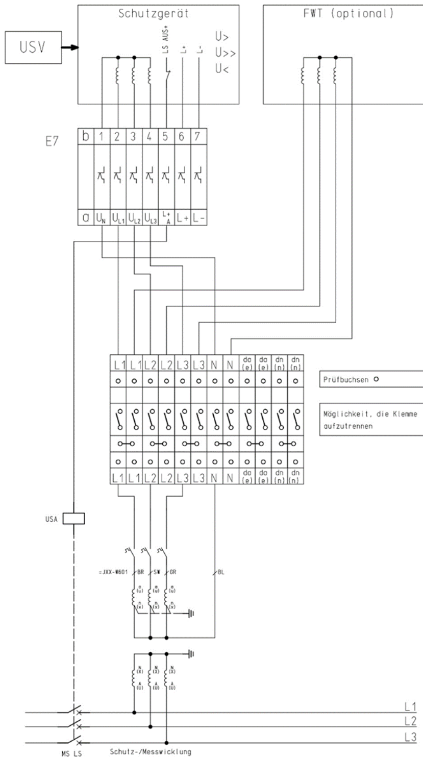
Abb. 46: Wandlerverdrahtung Anbindung übergeordneter Entkopplungsschutz / Fernwirkgerät
