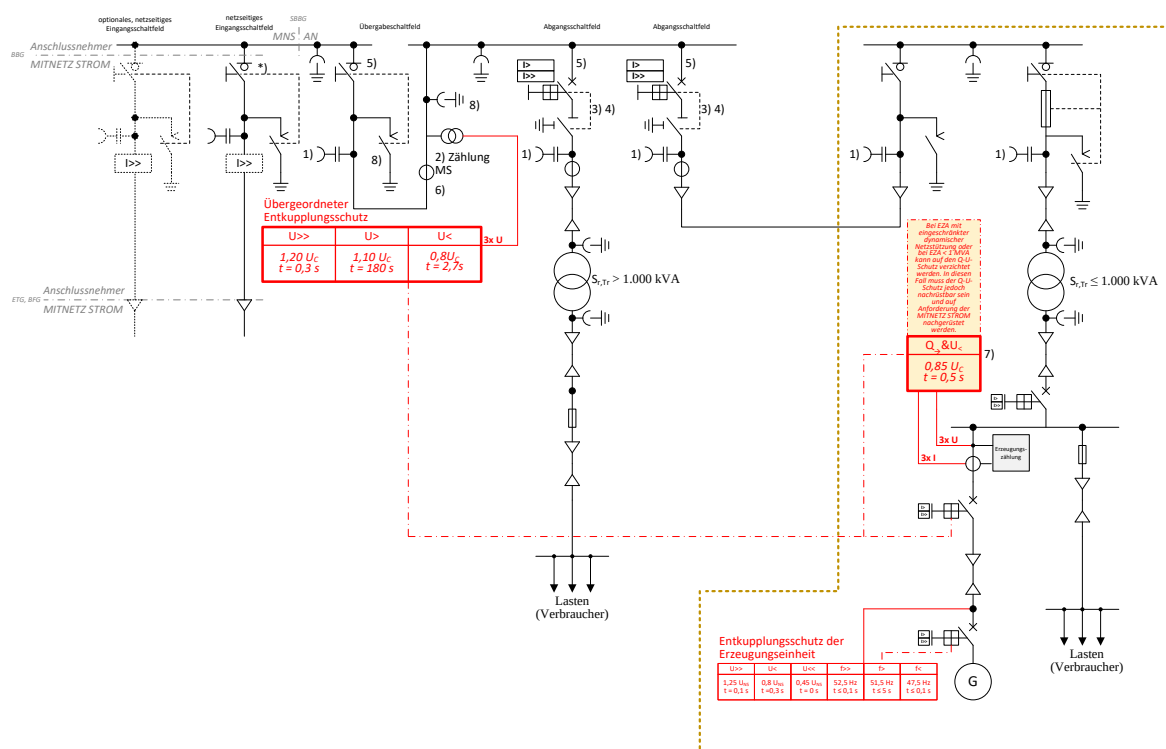
Abb. 33: (ehemals D5c): ≤ 20-kV-Anbindung einer Mischanlage mit nachgelagerter Station
