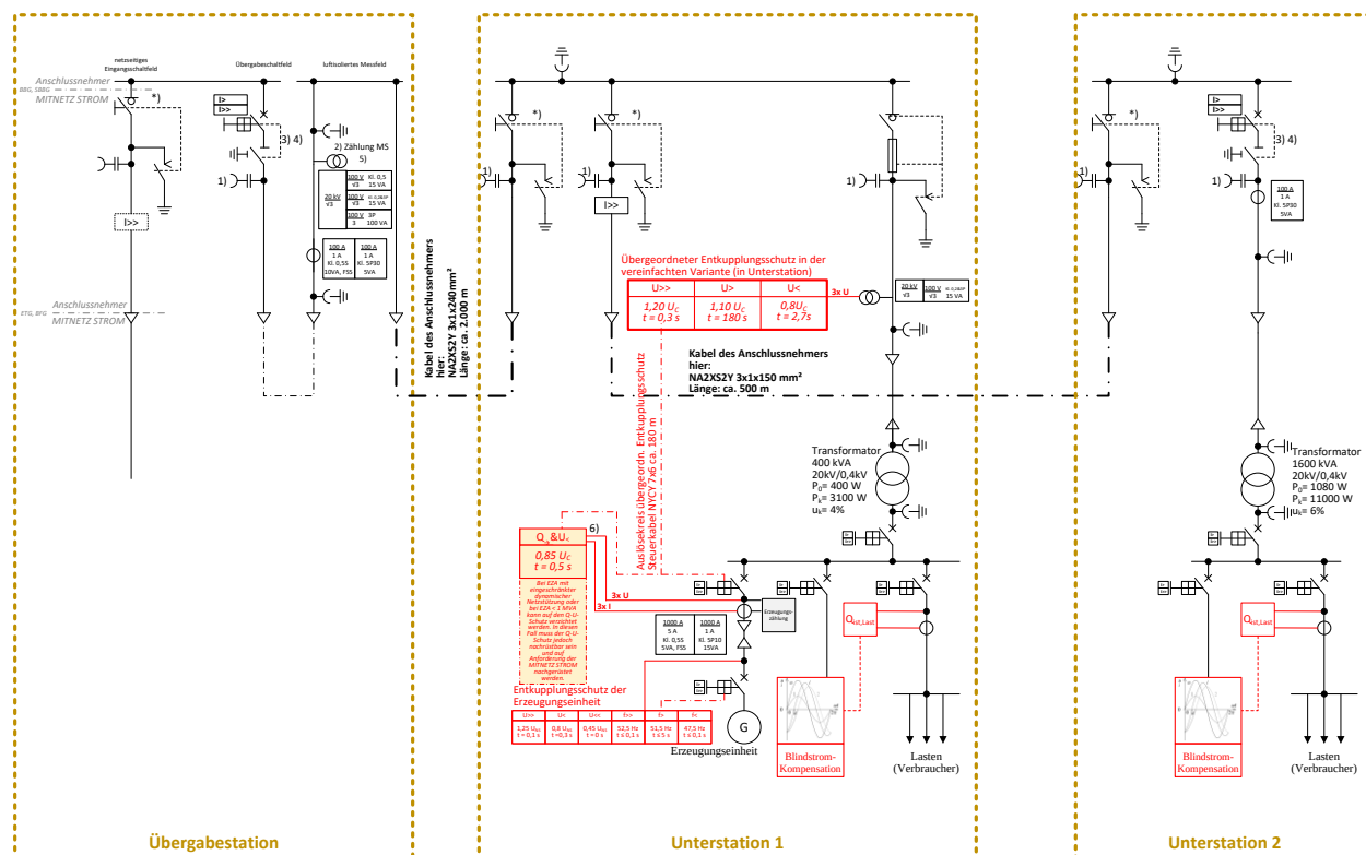
Abb. 35: (ehemals D5e): ≤ 20-kV-Anbindung von zwei Unterstationen mit Blindstromkompensation der Lasten der Bezugsanlage und vereinfachter Variante des übergeordneten Entkopplungsschutz
