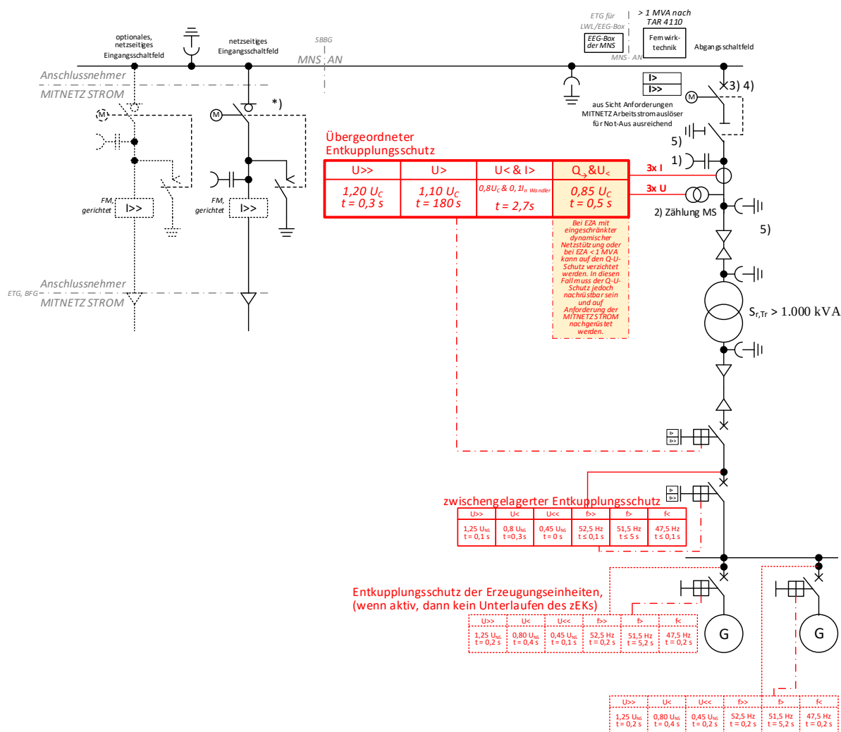
Abb. 29: (ehemals D4d): ≤ 20-kV- Anbindung einer Erzeugungsanlage &gt; 1 MVA
